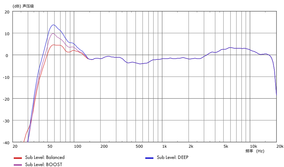
KC12 频率响应 (同轴, 1/3 倍频程平滑处理)
