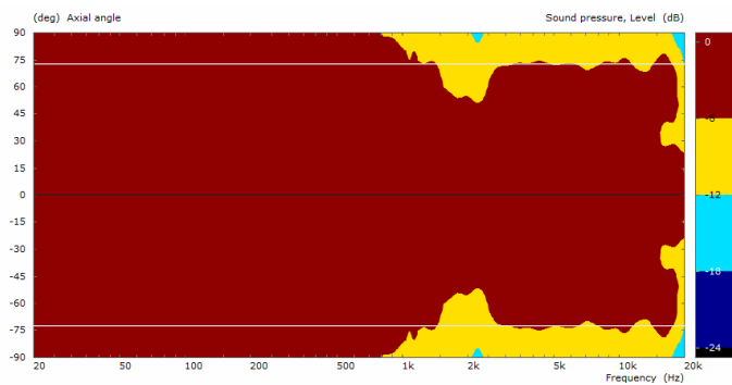
KC12 水平覆盖 (1/3 倍频程平滑处理)
