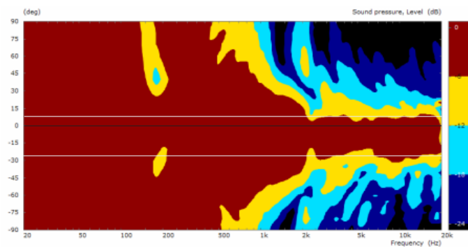
KC12 垂直覆盖 (高部署, 1/3 倍频程平滑处理)
