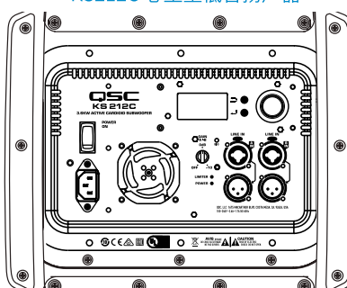
KS212C 心型重低音扬声器
